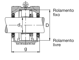
Vedação de feltro FSV
