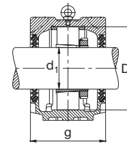
Vedação de dois lábios DH
