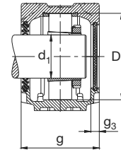
Vedação de dois lábios DH Tampa DKV
