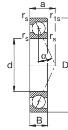
B719E, B70E, B72E Ângulo de contato \alpha = 25^\circ
