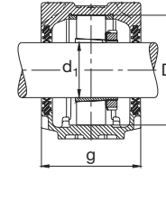
Vedação de dois lábios DH
