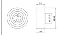
VKM 76202
