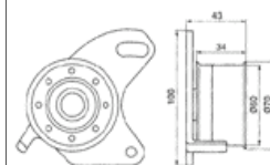
VKM 75601
